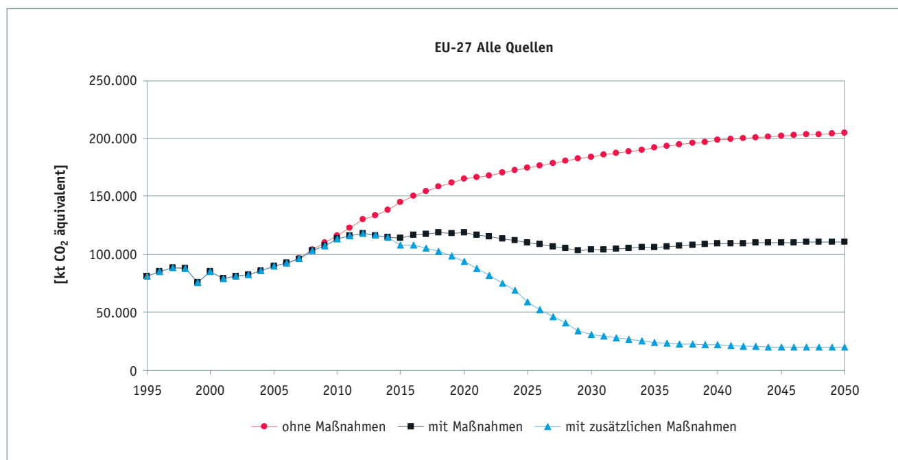
Abbildung 1: Berechnung der Minderung von F-Gas-Emissionen ohne Maßnahmen, mit bestehender Regulierung, mit ergänzender Regulierung (F-Gas Verordnung und MAC Direktive) (Quelle: Öko-Recherche 2011: Preparatory study for a review of Regulation (EC) No 842/2006 on certain fluorinated greenhouse gases)
